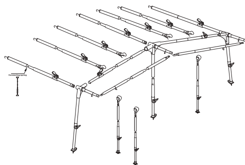
Armature PrenoX ORIANA Ø28 mm K10-N13
