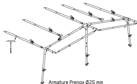
Armature PrenoX Ø25 mm Gb-K10
