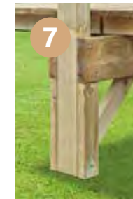
Jambe de force avant pour le poteau intermédiaire support charpente
